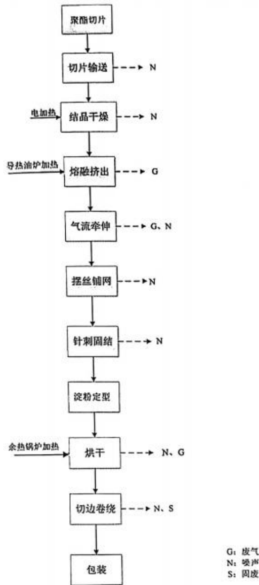
图 3 工艺流程图
